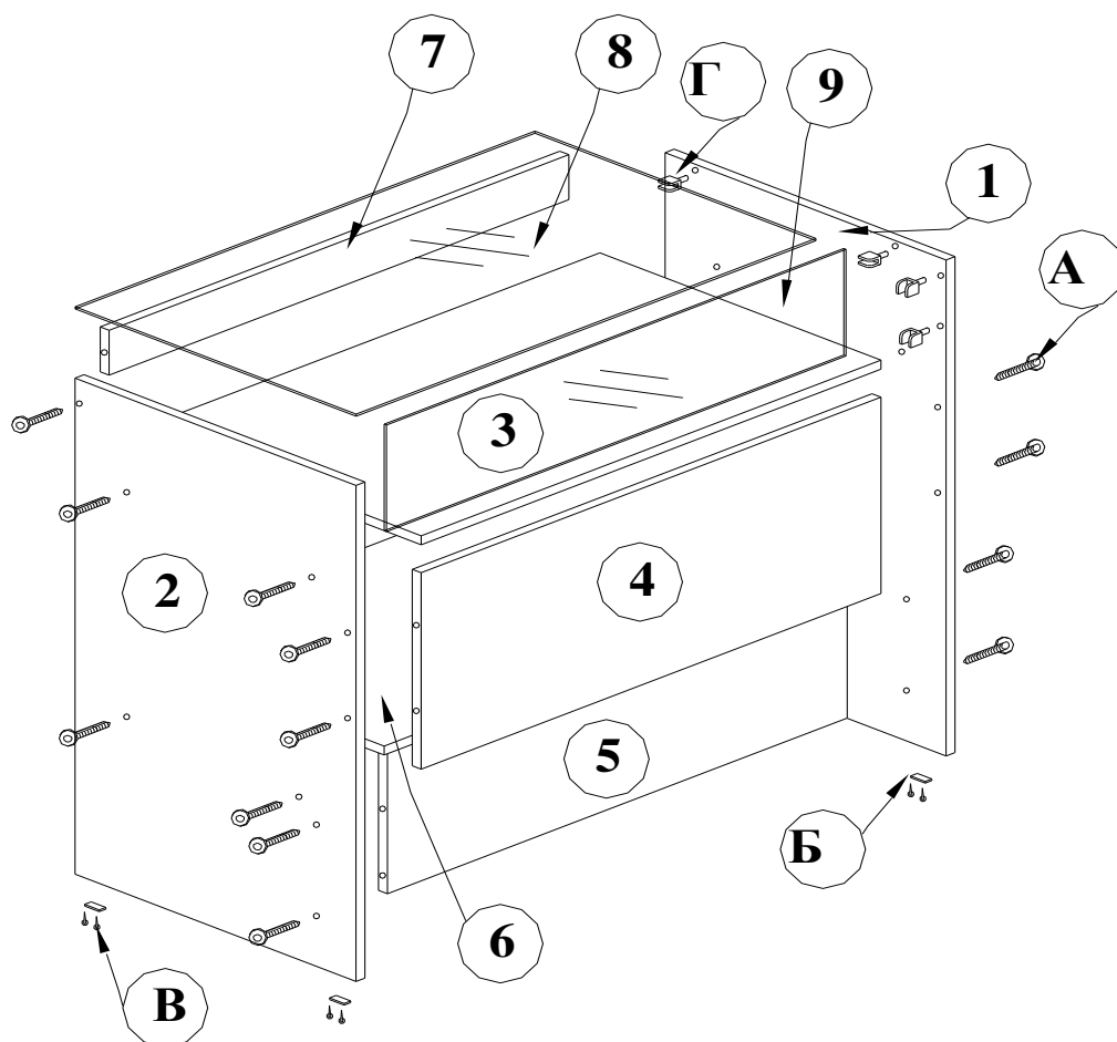
Пр-31 Прилавок остекленный малый 900x850x500
